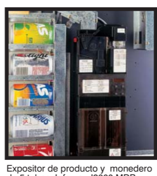
Expositor de producto y monedero de 5 tubos Jofemar J2000 MDB. Expositor do produto e porta-moedas de 5 tubos Jofemar J2000 MDB
