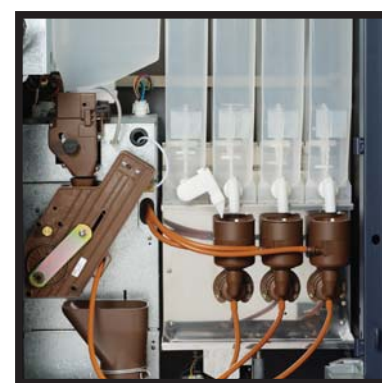
Detalle batidores y erogador G500 (Espresso) Wippers and brewer detail G500 (Espresso)
